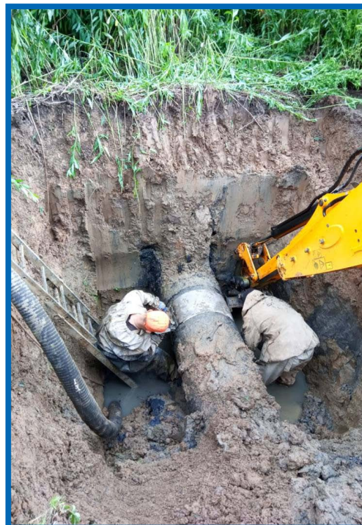
Установка ремонтного хомута мкр. Климовск, ул. Пролетарская, д.27
